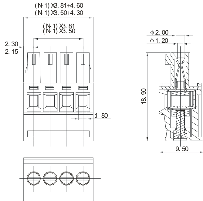
15EDGKA-3.5 15EDGKA-3.81
